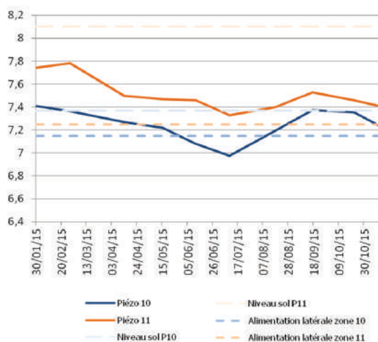
Suivi des niveaux d'eau dans la nappe des sables / niveaux NGF en m en 2015
