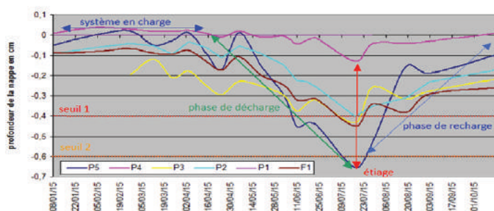
Evolution des niveaux de nappes en 2015
